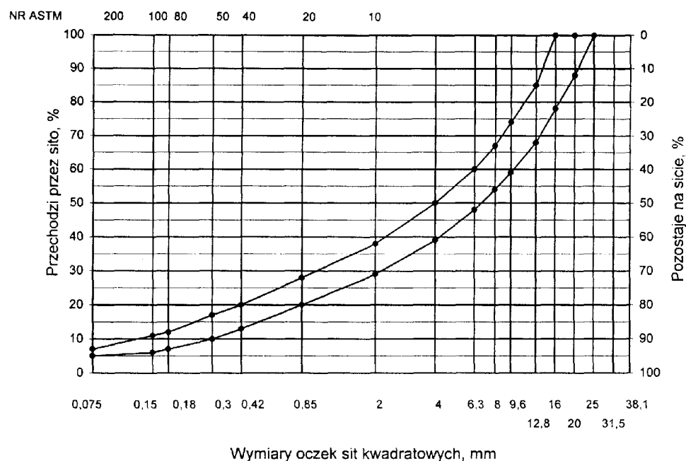
Rys. 4. Krzywe graniczne uziarnienia mieszanki mineralnej BA od 0 do 20 mm do warstwy ścieralnej nawierzchni drogi o obciążeniu ruchem KR3
